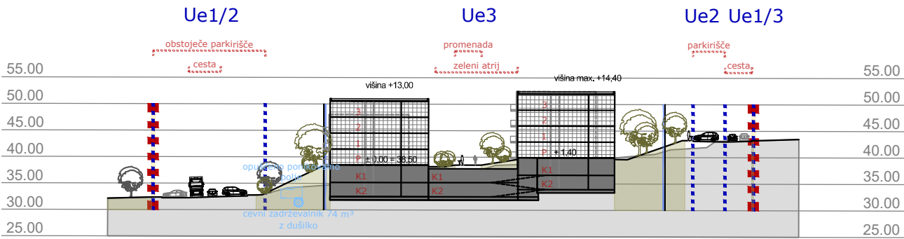
PREREZ 2-2
