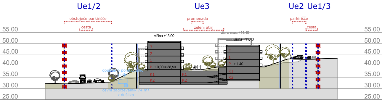
PREREZ 1-1
