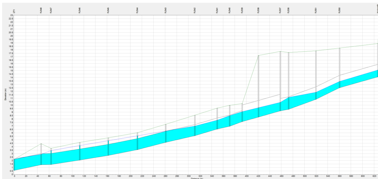
Slika 40: Vzdolžni profil kinete hudournika Ankanan z gladino Q_{100} – obstoječe stanje
