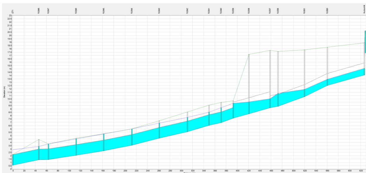
Slika 42: Vzdolžni profil kinete hudournika Ankaran z gladino Q 500 – obstoječe stanje
